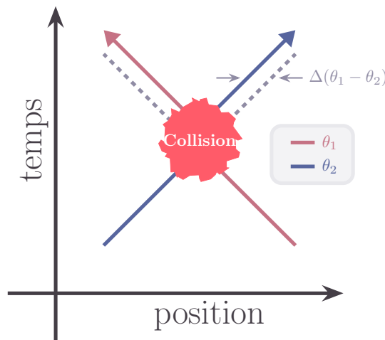
FIGURE 1.1 – Schéma de collision entre deux quasi-particules et du décalage spatial \Delta(\theta_1 - \theta_2) .
