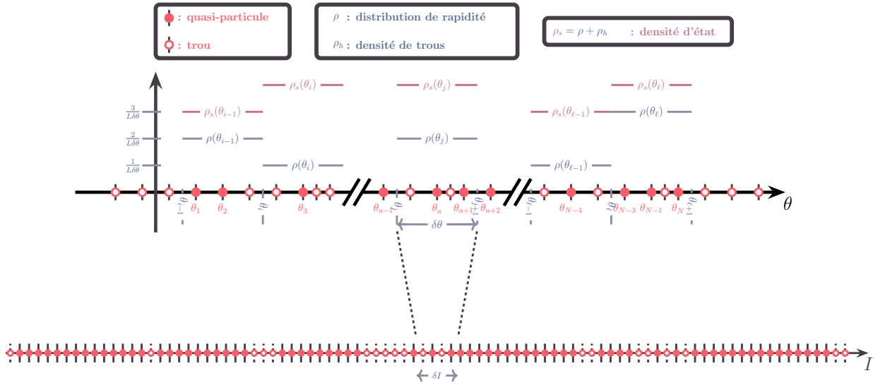
FIGURE 1.3 – Illustration de la relation entre la densité d'états \rho_s(\theta) et les nombres quantiques fermioniques I_a . Les rapidités dans l'intervalle [\theta, \theta + \delta\theta] s'associent à un ensemble de nombres quantiques fermioniques situés dans [I, I + \delta I] . La densité d'états \rho_s se déduit alors de la relation \delta I \simeq L\rho_s(\theta)\delta\theta
